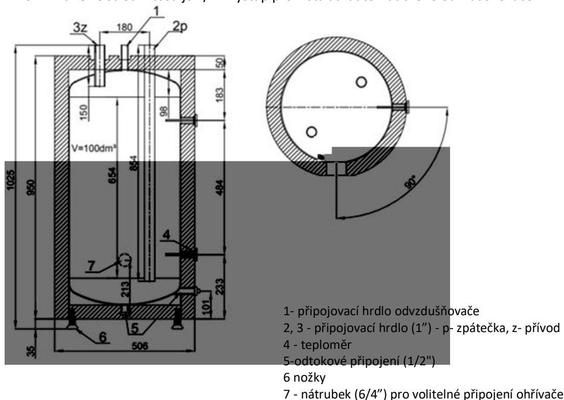
Obr. 1 Schéma vyrovnávací paměti BME 100. Obr
